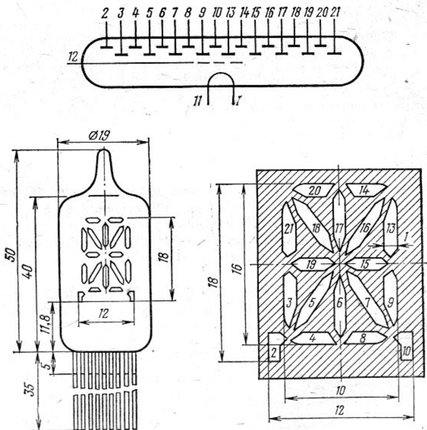
Расположение и условное обозначение анодов-сегментов ИВ-4
