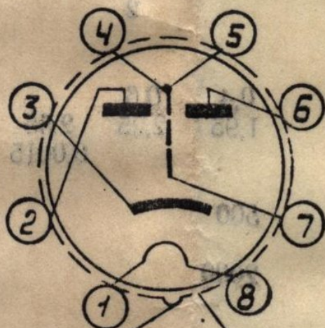
Схема соединения электродов лампы со штырьками
