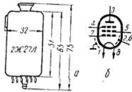
Рис. 94. Лампа 2Ж27Л:
