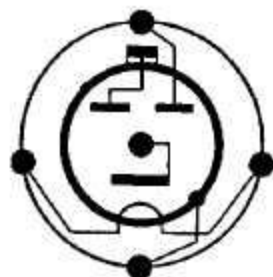
Sockelschaltung
