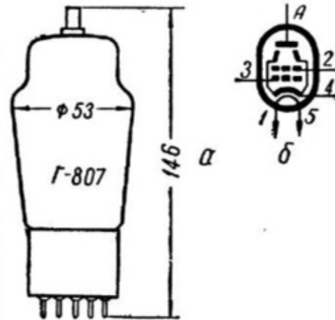
Рис. 559. Лампа Г-807:
