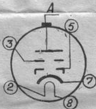
Расположение штырьков РШ 5-1 ГОСТ 7842—71
