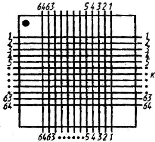
Схема соединения электродов с выводами
