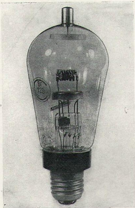
Внешний вид лампы ВГ-129
