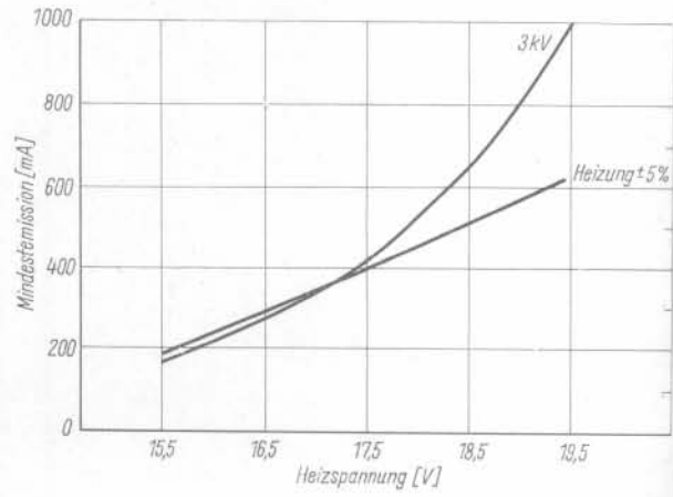
Emissions- und Heizcharakteristik: Gemessen bei 3 kV kk-Gleichspannung
