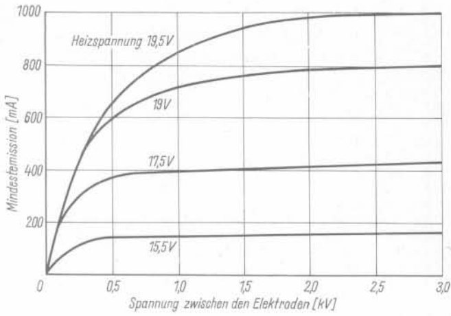
Emissionscharakteristik:
