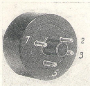
Вид на лампу 0,3Б65-135 снизу
